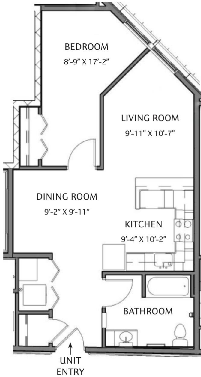
TYPE 4 - 1 BEDROOM
