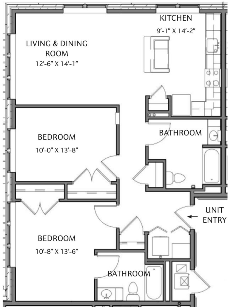
TYPE 3 - 2 BEDROOM
